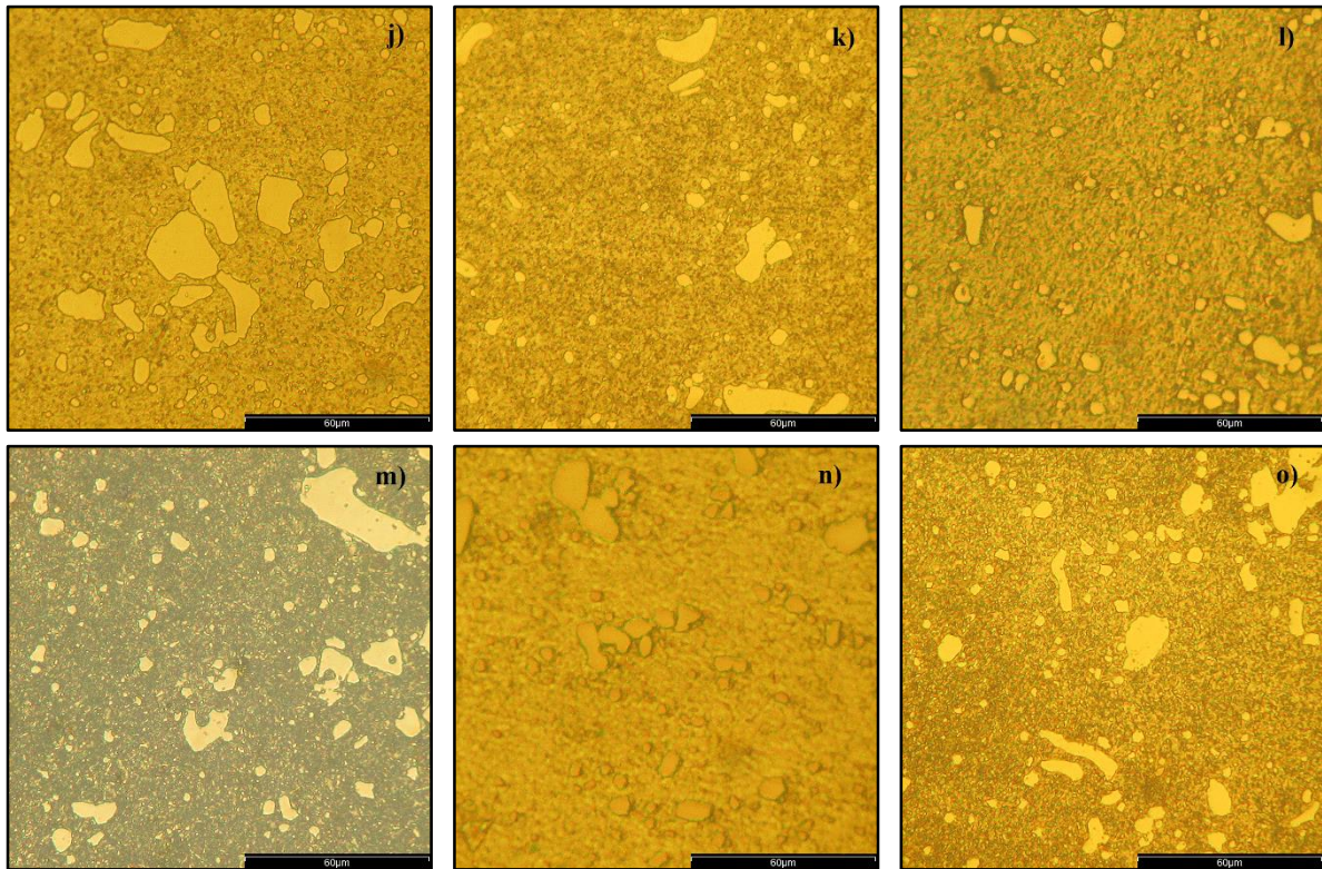
Figure 5. Microphotographs of the samples after: a) quenching; and after tempering at: b) 50 °C; c) 100 °C, d) 150 °C, e) 200 °C, f) 250 °C, g) 300 °C, h) 350 °C, i) 400 °C, j) 450 °C, k) 500 °C, l) 550 °C, m) 600 °C, n) 650 °C, o) 700 °C; magnification \times 1000
